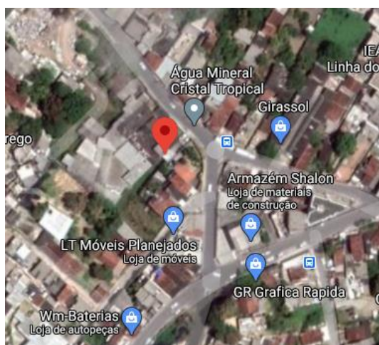
Contexto local
